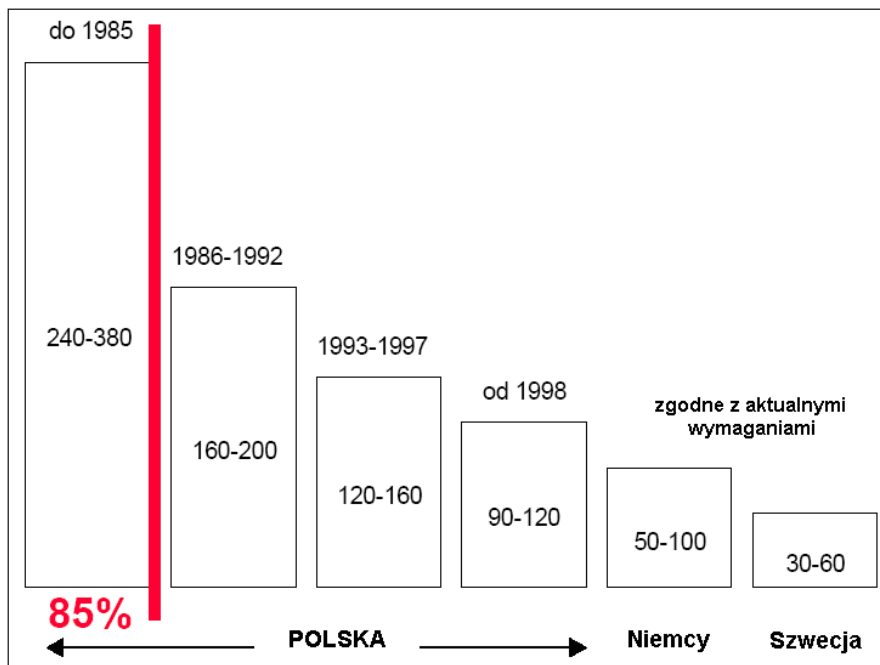
Rys.1. Średnie zużycie ciepła na cele grzewcze w kWh/m² powierzchni użytkowej Źródło: Instytut Budownictwa Pasywnego www.pibp.pl
