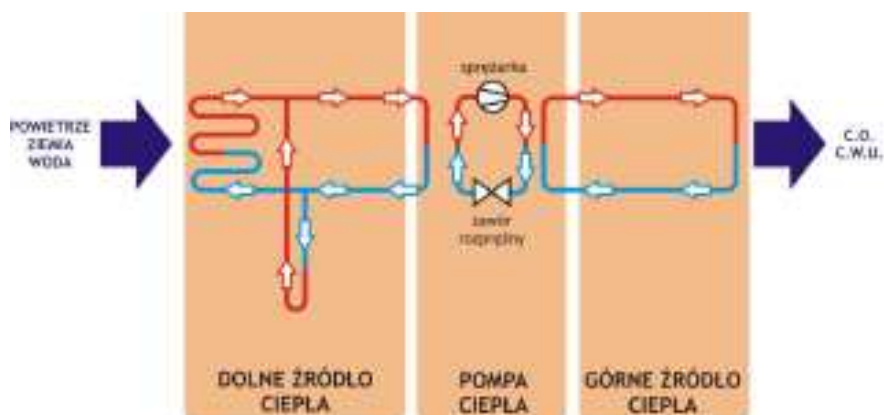
Rys. 4. Zasada działania pompy ciepła Źródło: Instytut Energetyki Odnawialnej (EC BREC IEO)
