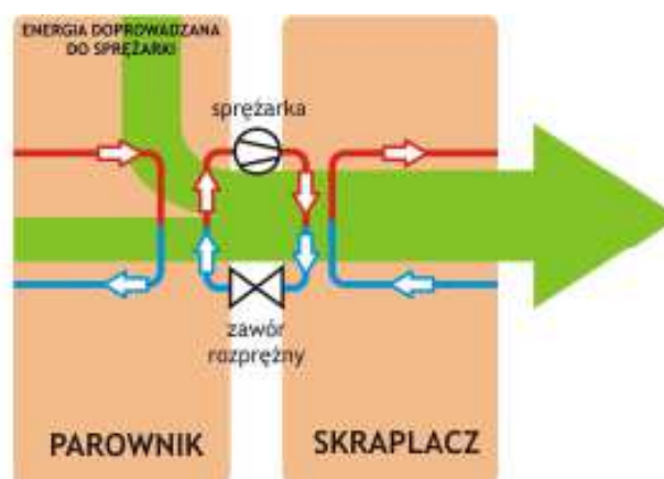
Rys.5. Obieg pośredni pompy ciepła Źródło: Instytut Energetyki Odnawialnej (EC BREC IEO)
