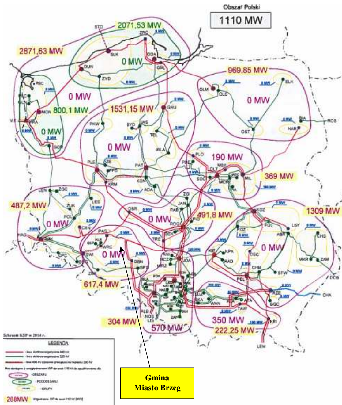
Rys.4. Schemat sieci przesyłowej z dostępnymi mocami przyłączeniowymi – stan wyjściowy na rok 2014 Źródło: http://www.pse.pl
