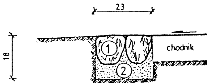
Rys. 1. Obramowanie chodnika z brukowca od 10 do 12 cm
