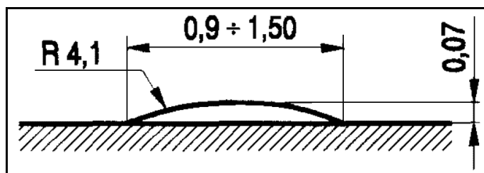
Rys. 4. Przekrój podłużny liniowego progów zwalniającego listwowego o ograniczonej prędkości przejazdu 18 ÷ 20 km/h (U-16d)
