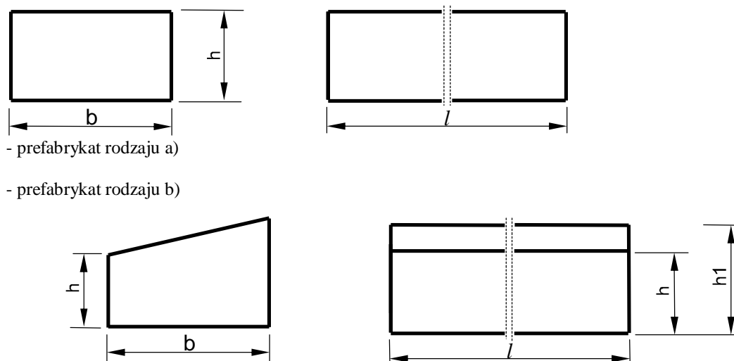
Rys. 7. Wymiarowanie prefabrykatów
