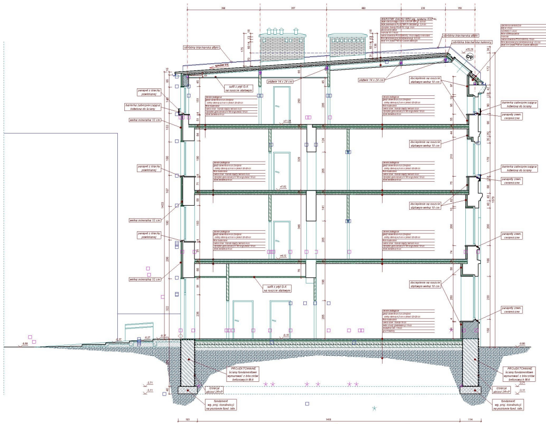
BRUKI: w przedmiotowych miejscach bruków i kostki zastosować Ecolife z S&B z wyjątkiem dla ścieżki max. 20 cm. RYSLINKI PROJEKTU ARCHYTEKTONICZNEGO ROZPATRYWAĆ ŁĄCZNIE Z PROJEKTAMI BRANŻOWYMI
