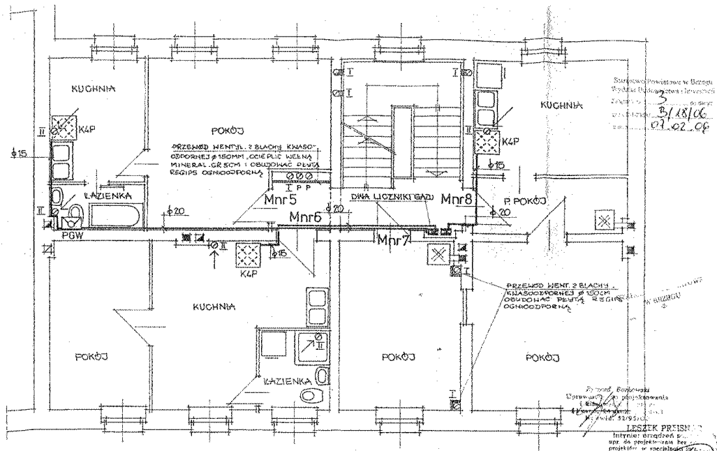
rzut II-go piętra skala 1:50 projekt instalacji gazu
