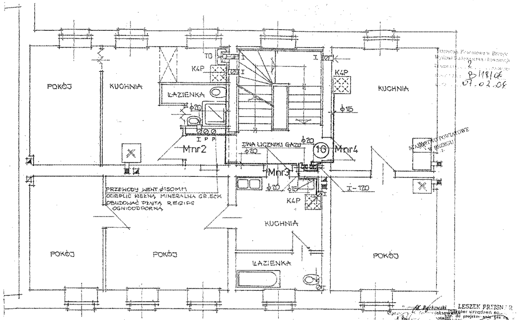
rzut I-go piętra skala 1:50 projekt instalacji gazu
