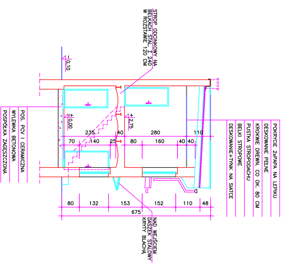
PRZEKRÓJ POPRZECZNY A-A
