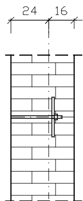
Usytuowanie pręta ściagu S4 w murze /1:20/
