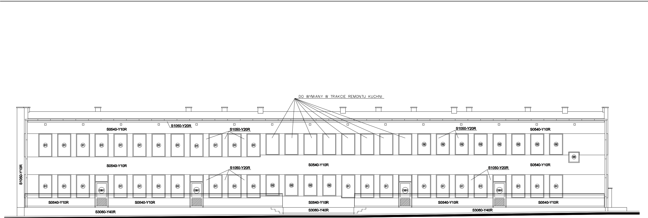
ELEWACJA WSCHODNIA 1:100
