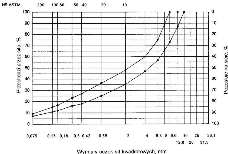
Rys. 1. Krzywe graniczne uziarnienia mieszanki mineralnej BA od 0 do 12,8 mm do warstwy ściernalnej nawierzchni drogi o obciążeniu ruchem od KR3 do KR6
