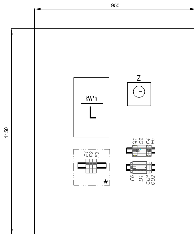
widok wyposażenia szafki złączowo-pomiarowej oświetlenia drogowego w obudowie ZKW
