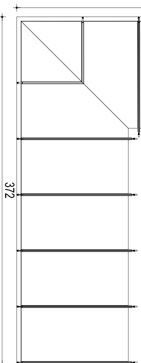
DASZEK POLIWĘGLANOWY TYP 1
