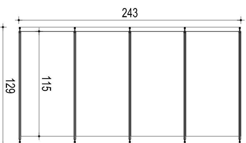
DASZEK POLIWĘGLANOWY TYP 2
