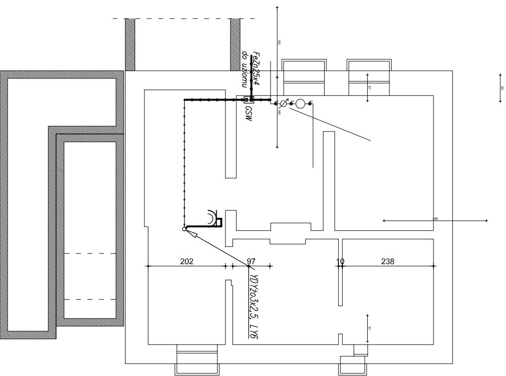
RZUT PIWNIC
