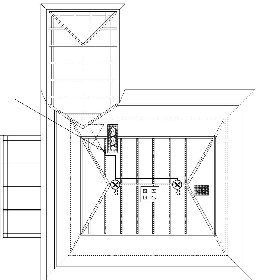
RZUT PODDASZA
