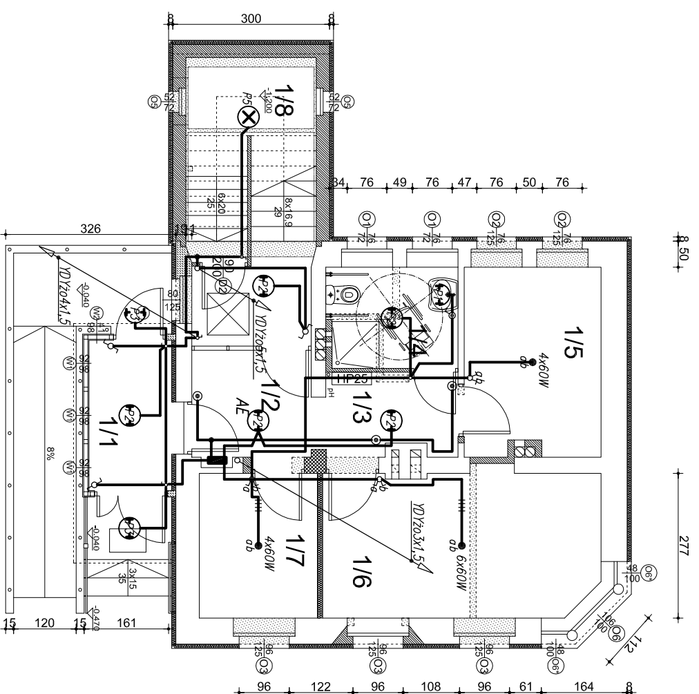
RZUT PARTERU
