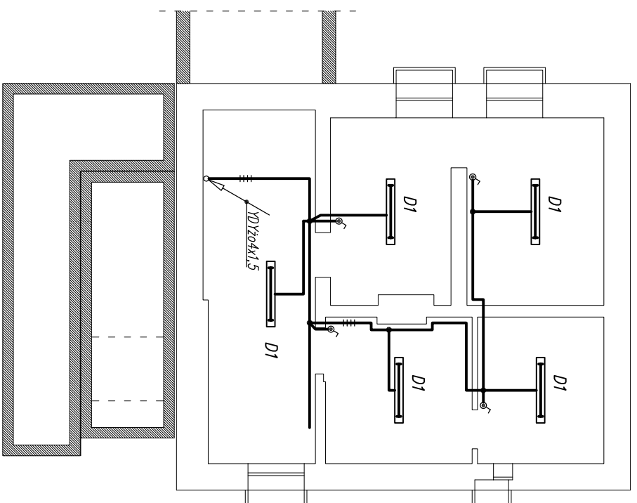
RZUT PIWNIC
