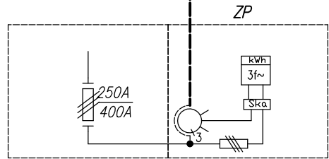
Skrzynka złączowo-pomiarowa wykonanie i własność EnergiaPro
