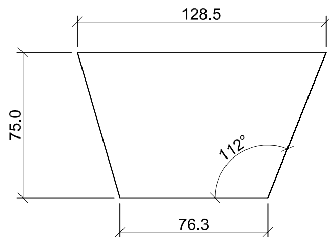
WIDOK 3
