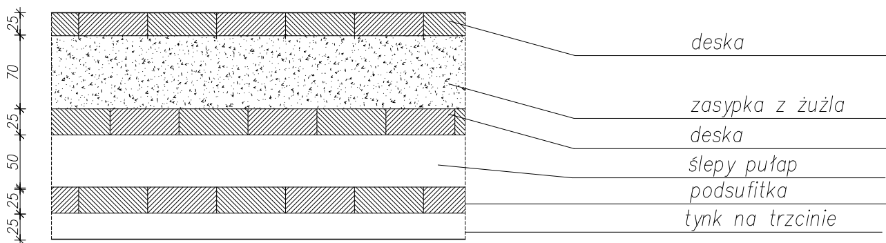
Przekrój B
