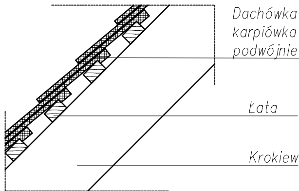
Przekrój B
