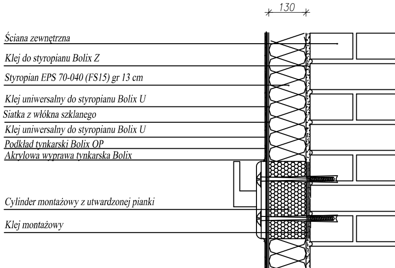
Detal mocowania elementów zewnętrznych
