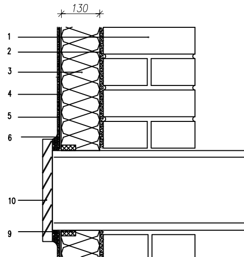
Ocieplenie w obrębie połączenia z kratką wentylacyjną stropodachu
